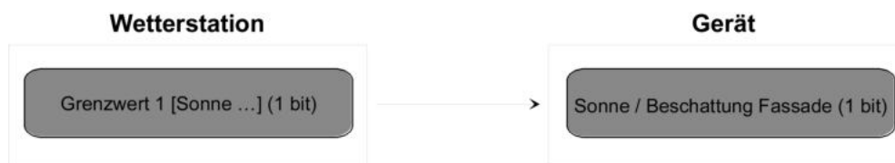
Bild 28: Projektierung der Kommunikationsobjekte für Anwendungsbeispiel I.
