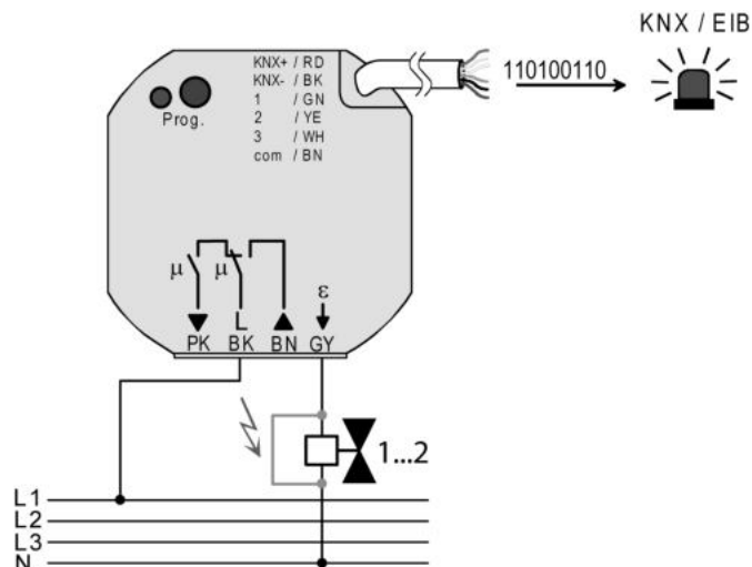
Bild 52: Kurzschluss- und Überlasterkennung bei Störung des Ventilausgangs oder Ventiltriebs
