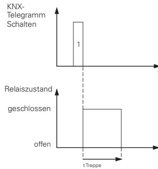
Treppenlichtzeitfunktion
