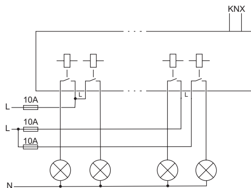
Bild: Anschlussbeispiel
