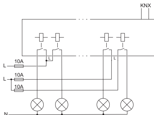
Bild: Anschlussbeispiel
