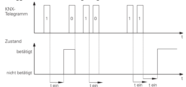
Retriggerbare Einschaltverzögerung
